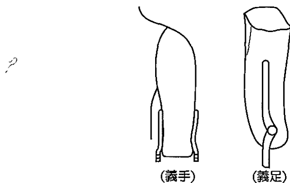
図-8 支持部を加算できないソケット
