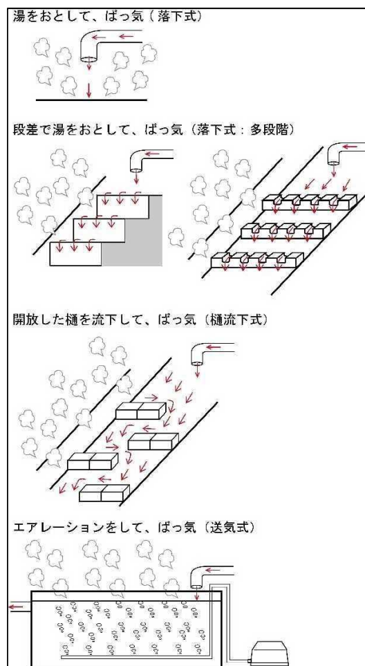
図3 ばっ気装置概念図
