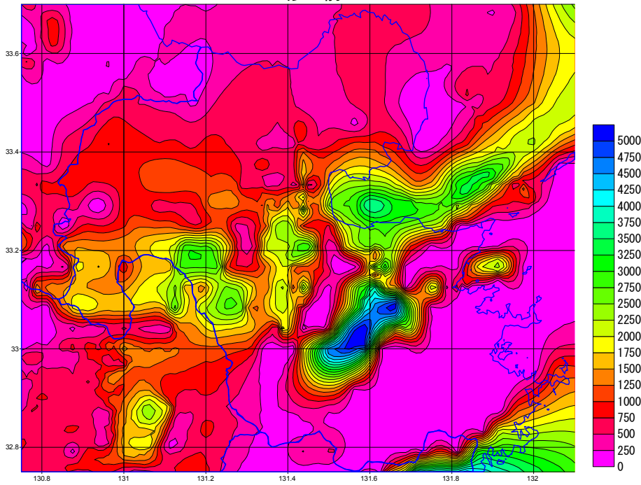
図 2-3-9 第 5 層 (Vs3.1) 上面深度コンター
