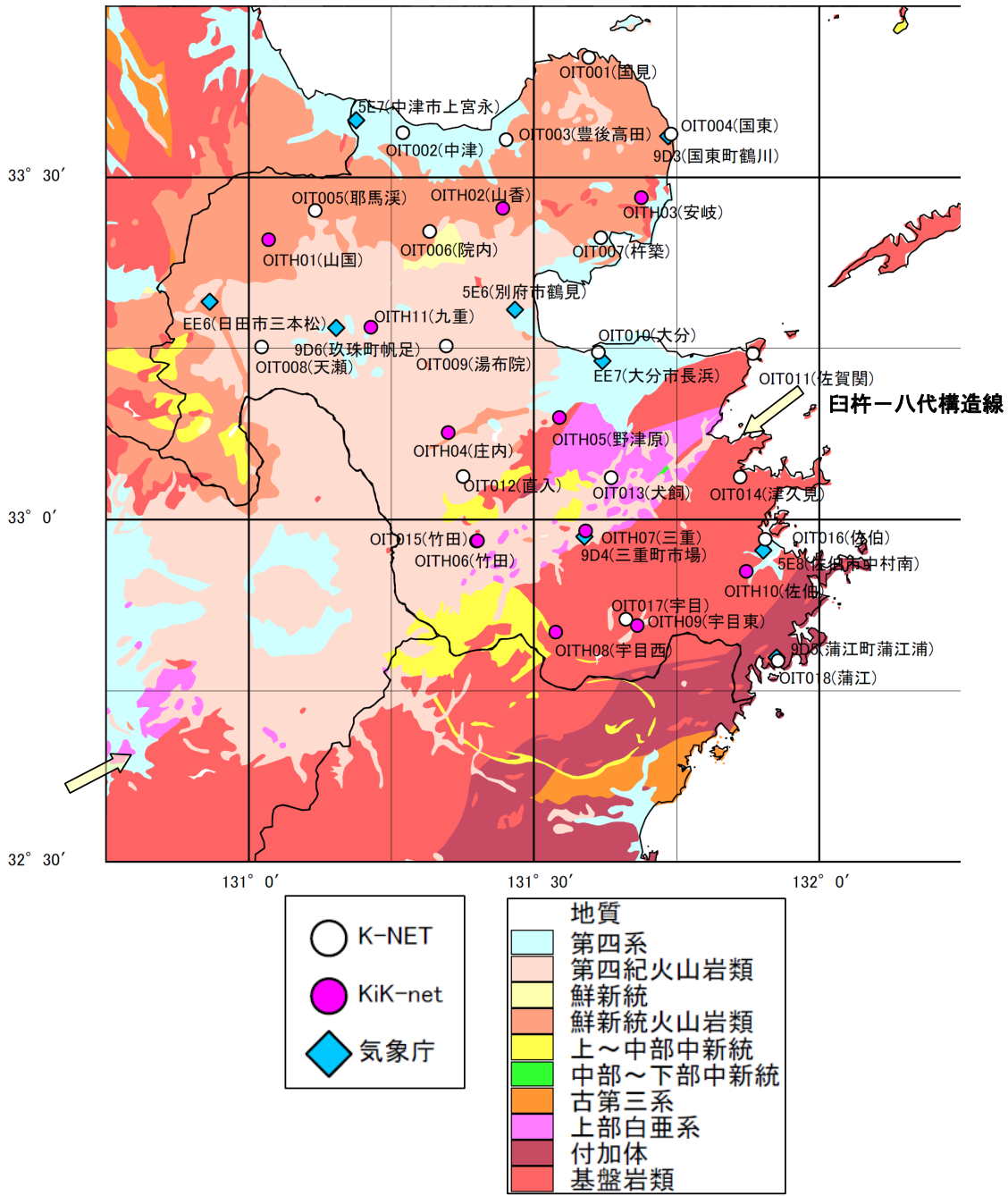
図2-1-1 大分県内の地質分布図とモデル作成に用いた地震観測地点の位置 産業技術総合研究所のシームレス地質図をトレースして作成。
