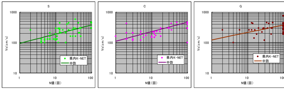
図 2-4-2 N 値と Vs の関係 (県内 K-NET より)
