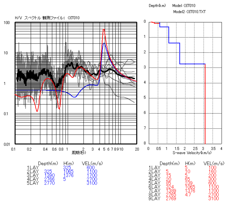
図 2-3-13 OIT010 地点の理論H/Vスペクトル
