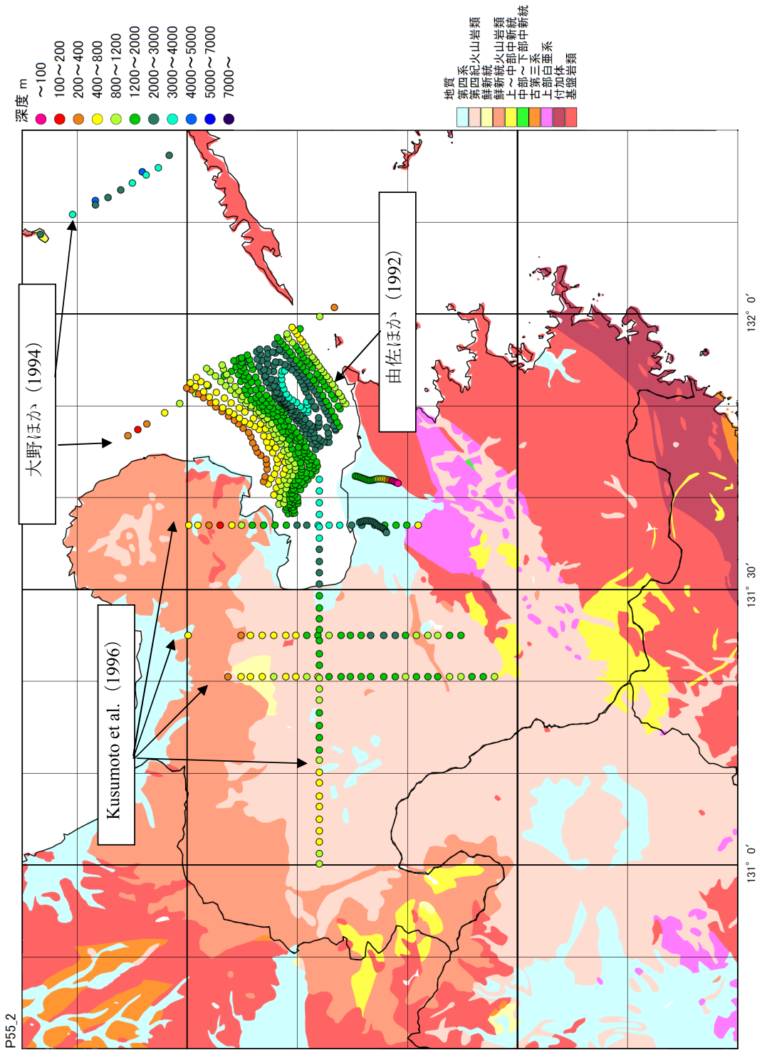
図 2-3-1 大分県の地質図と物理探査データの位置 (地震 hypocenter 深度を深さに応じて色分けして表示)
