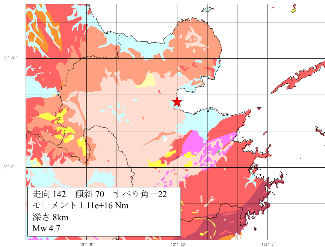
図 2-3-11 2007 年 6 月 6 日 23 時 42 分 大分県中部の地震の震央位置 (震央位置は気象庁速報による)
