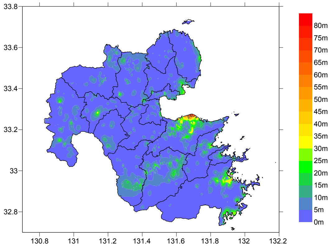
図 2-4-3 工学的基盤コンター
