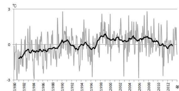
図5. 1980～2013年気温の月別偏差・25ヵ月移動平均の推移（豊後高田市）
