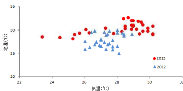
図18. 2012・2013年8月の長洲C1における地温(満潮時)と豊後高田市気温との関係
