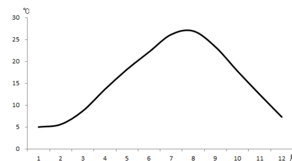
図3. 1980～2013年気温の月別平年値（豊後高田市）
