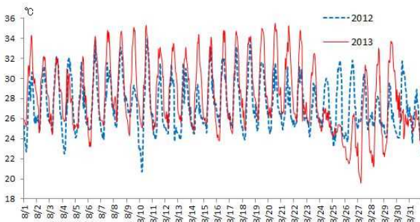
図8. 2012・2013年8月の気温の経時変化(豊後高田市)
