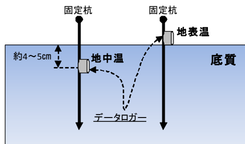
図2. データロガー設置位置の模式図
