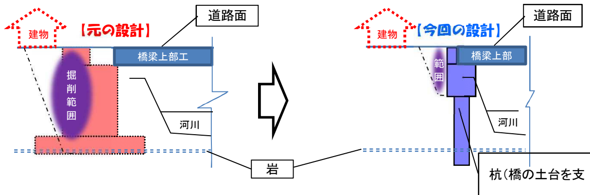
橋の土台の比較図(イメージ図)
