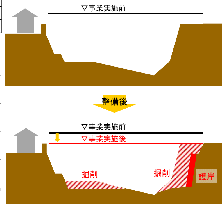
●整備後の状況
