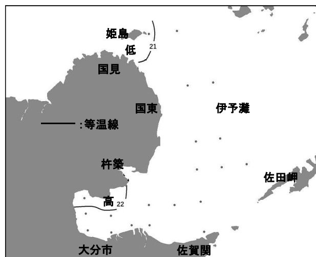
30m層水温分布
