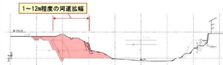
横断面図
