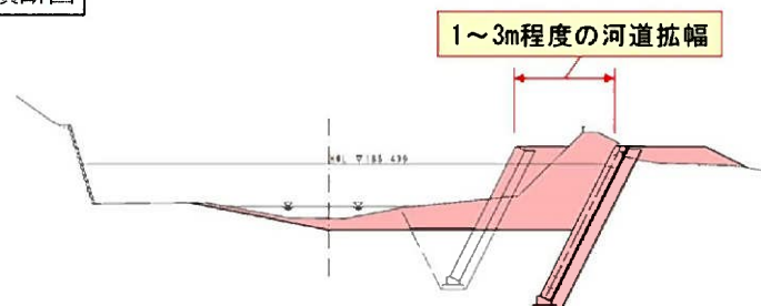
横断面図
