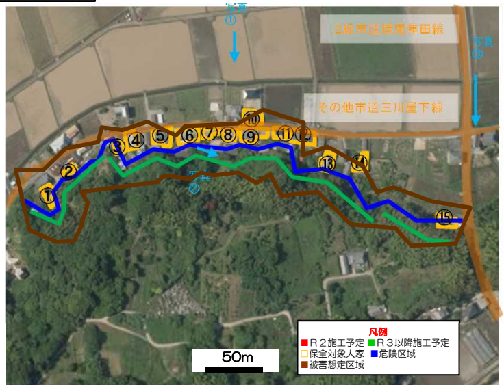
全景
