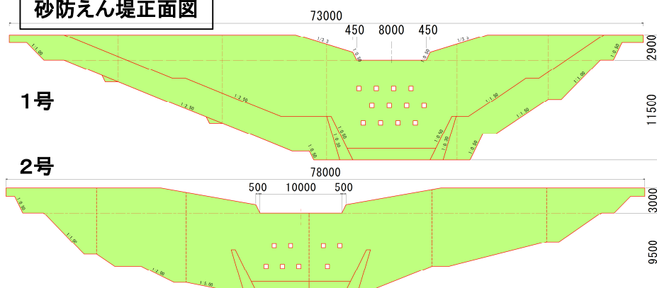
砂防えん堤正面図
