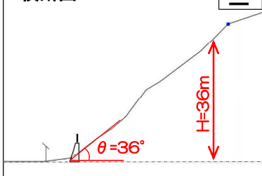
横断面図
