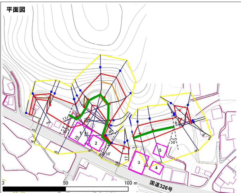
斜面状況
