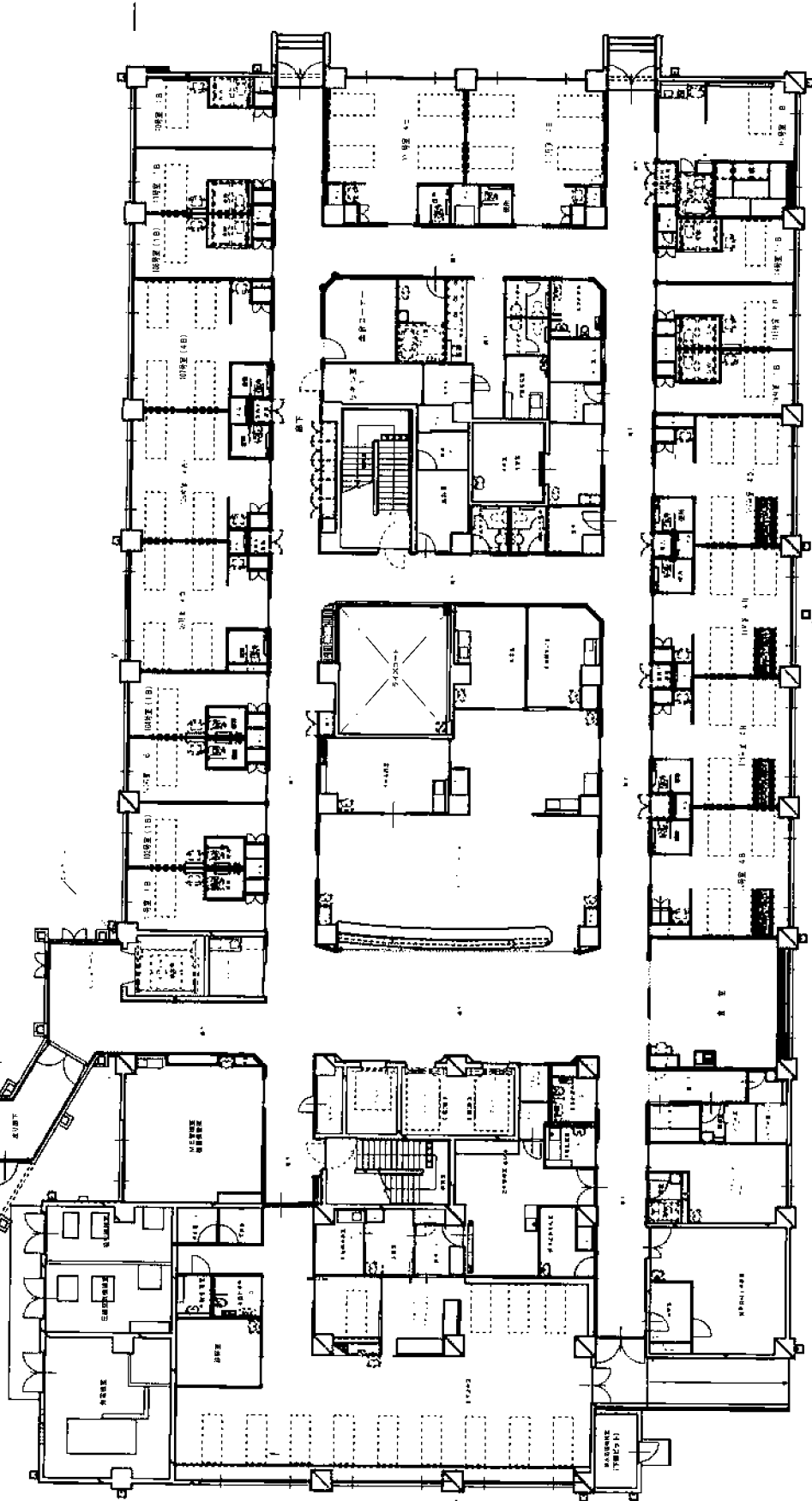
1 隨平面圖
