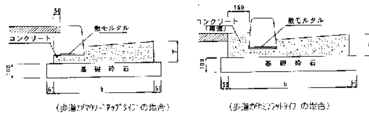
図 13-1 側溝及び街渠参考図（単位：mm）
