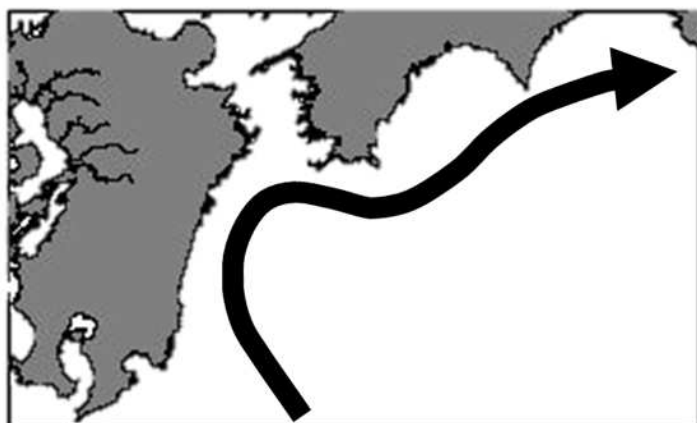
黒潮流路図
