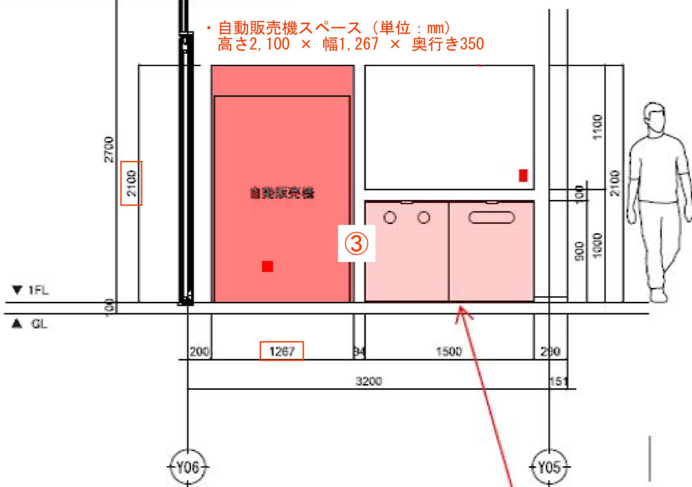
展開図
