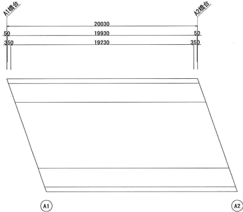
平面図 S=1/100
