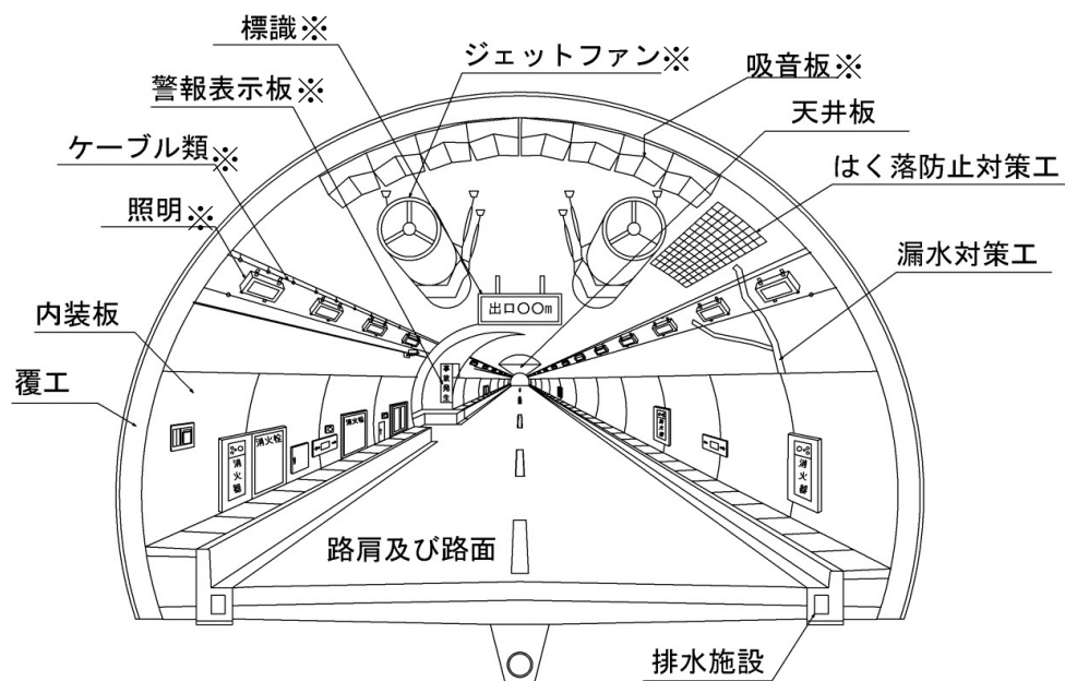
図－解 3.4 標準的な点検対象箇所（トンネル内）
