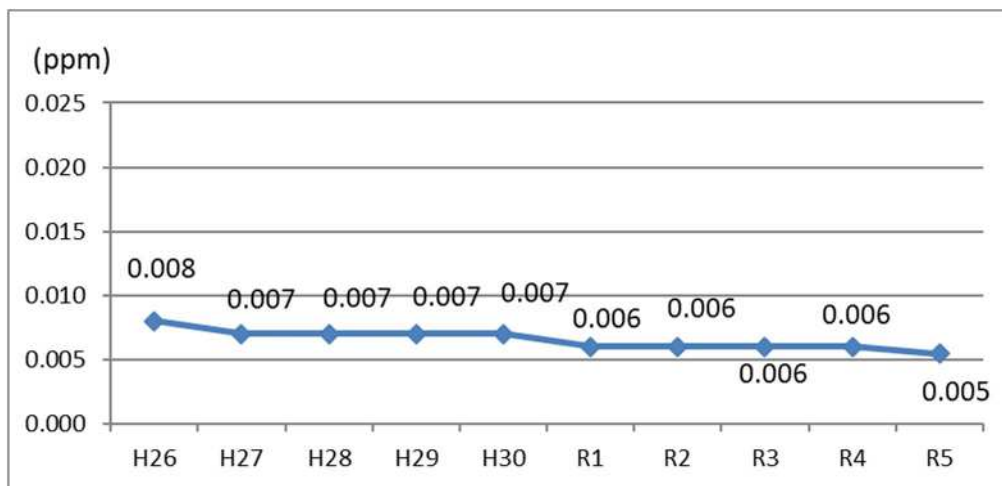
図 1-1-2(a) 二酸化窒素に係る年平均値の経年変化(一般環境大気測定局)
