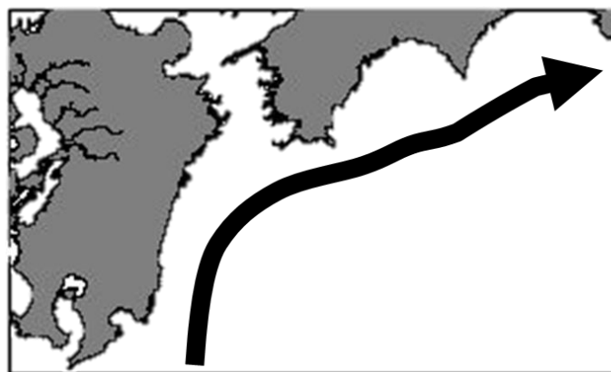
黒潮流路図
