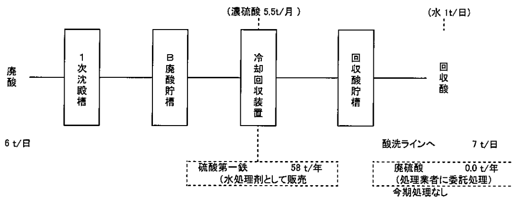
図2 廃酸回収フローシート
