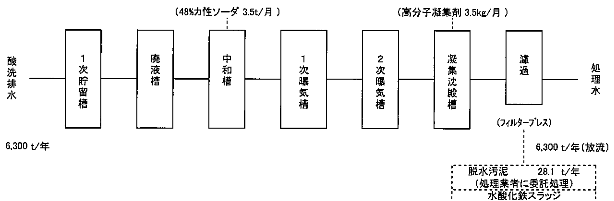
図3 排水処理フローシート
