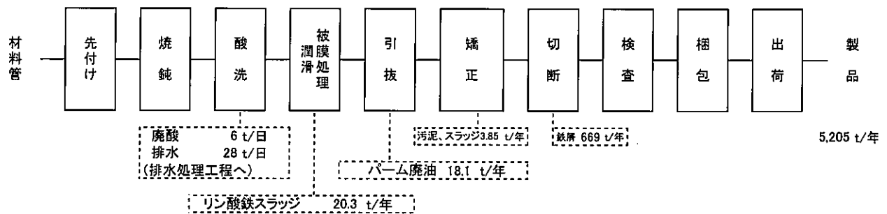
図1 冷間引拔鋼管製造フローシート
