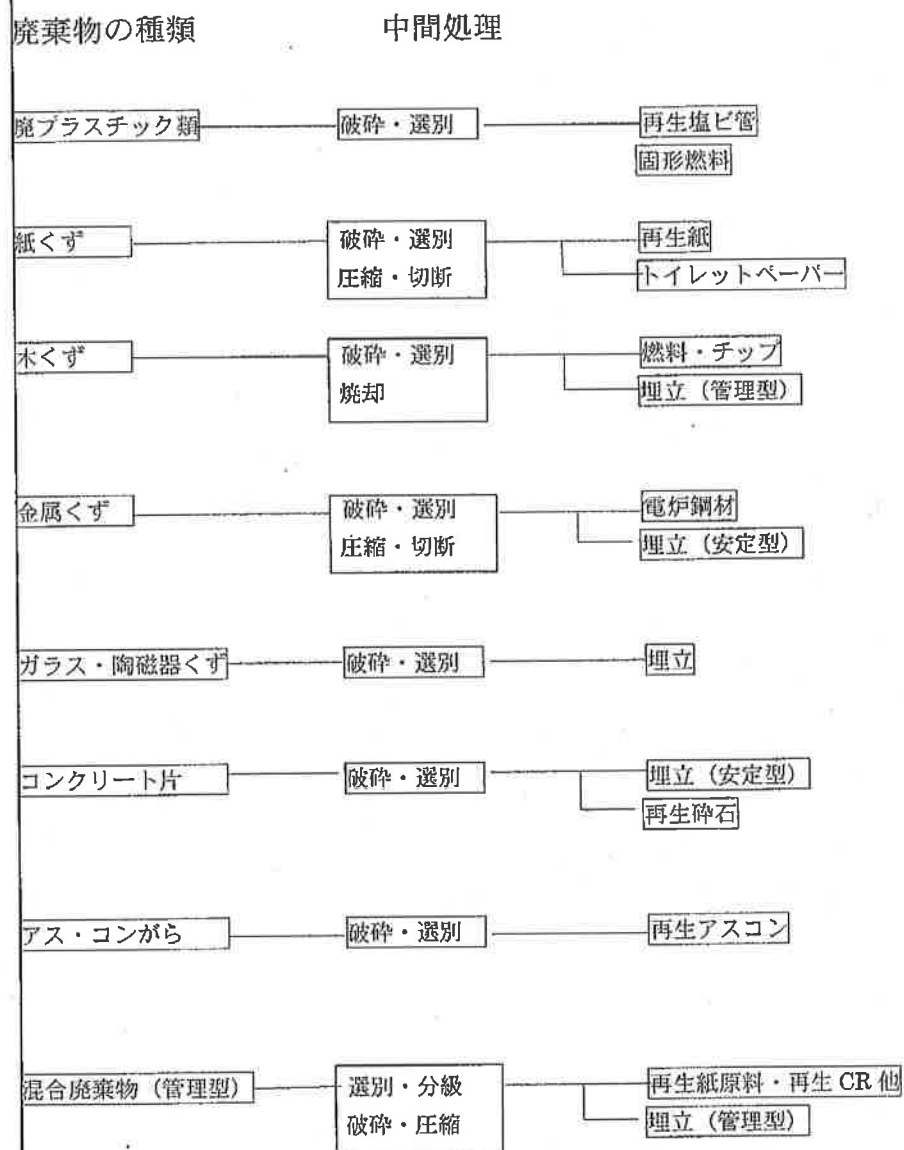
(別添 1) 産業廃棄物処理フロー図
