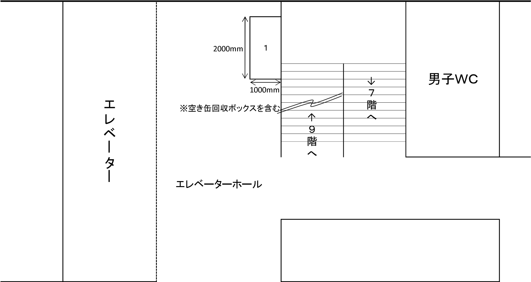
県庁舎本館8階自販機コーナー 貸付予定位置詳細図1
