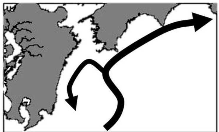
黒潮流路図
