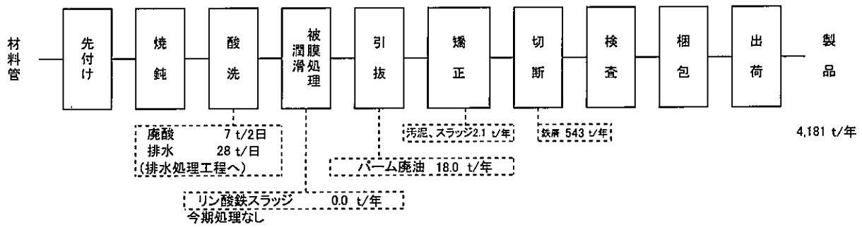
図1 冷間引抜鋼管製造フローシート
