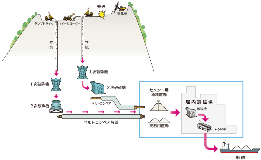
鉱山 模式図
