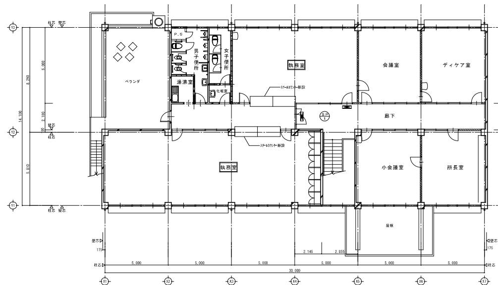
改修 2 階平面図 S=1/100
