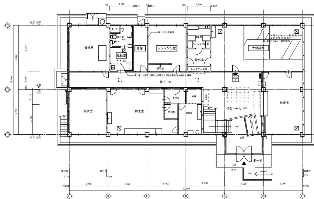
改修1階平面図 S=1/100 ・・・改修室を示す。
