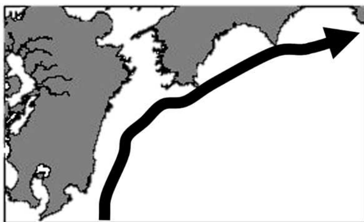
黒潮流路図
