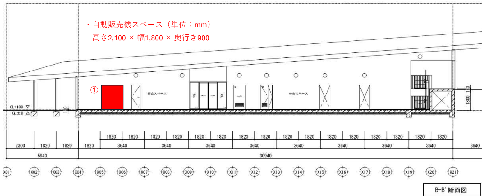
断面図
