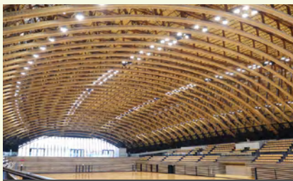
昭和電気武道スポーツセンター 木材を使った国内最大級のトラス構造
