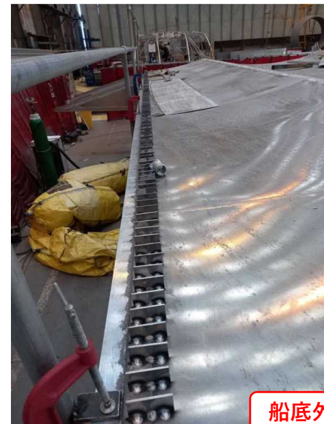
船尾端機関室底部構造
