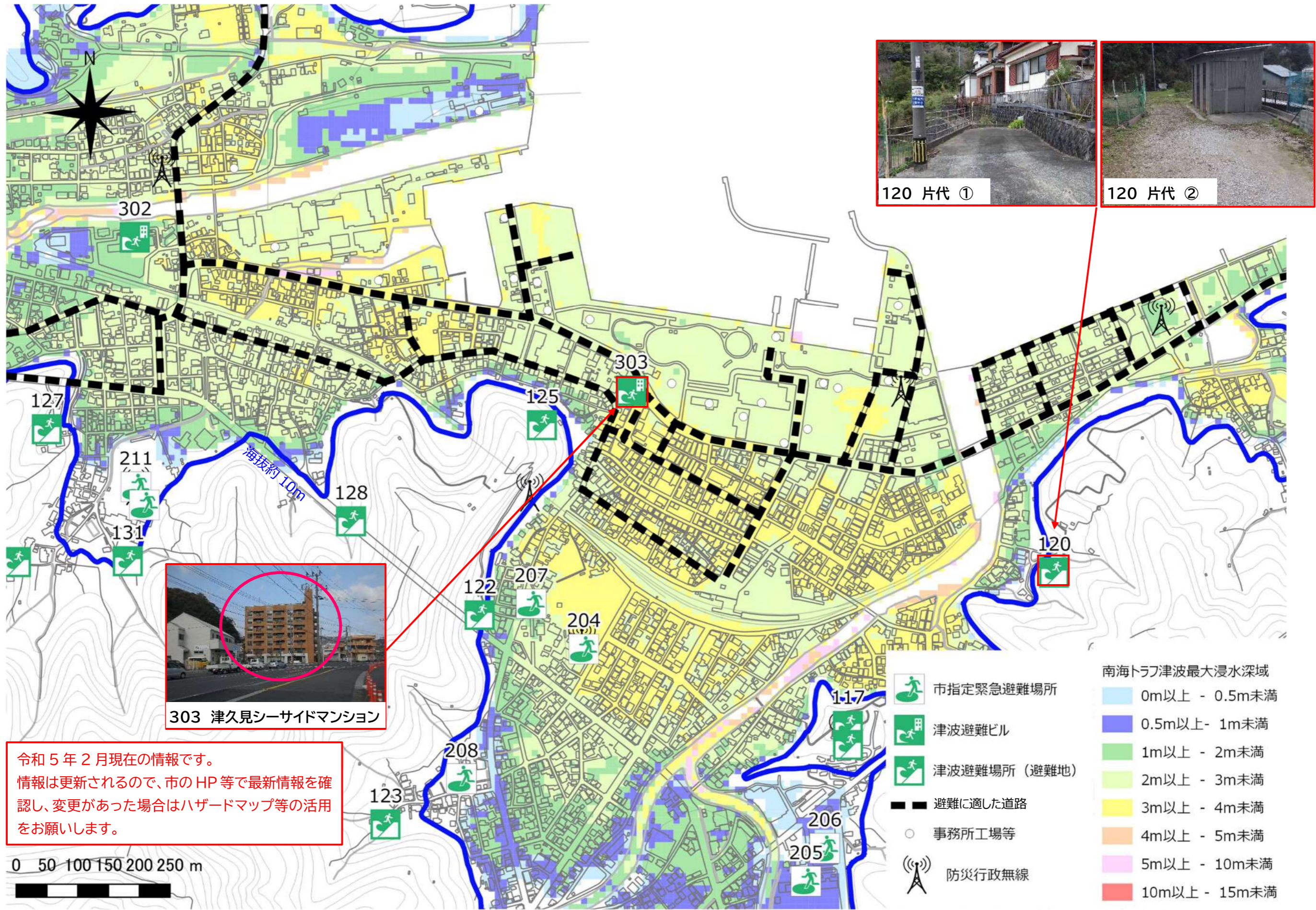
図 5-2 避難経路等と避難施設等の参考例 津久見港 港湾津波避難計画 港湾地域【F】 P12
