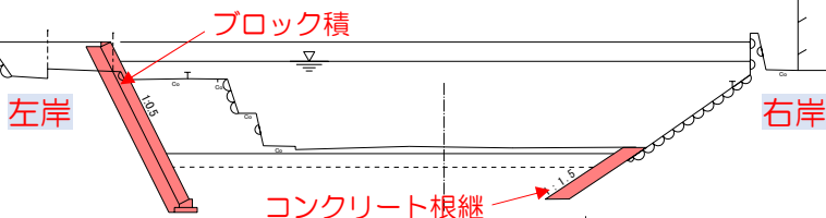
(B-B断面)
