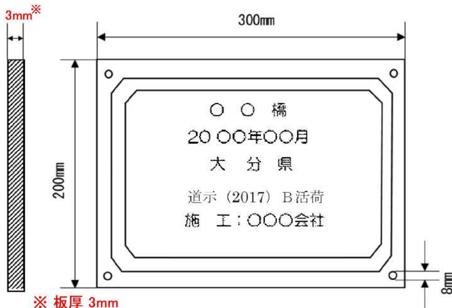
図 2－2 銘板の寸法及び記載事項
