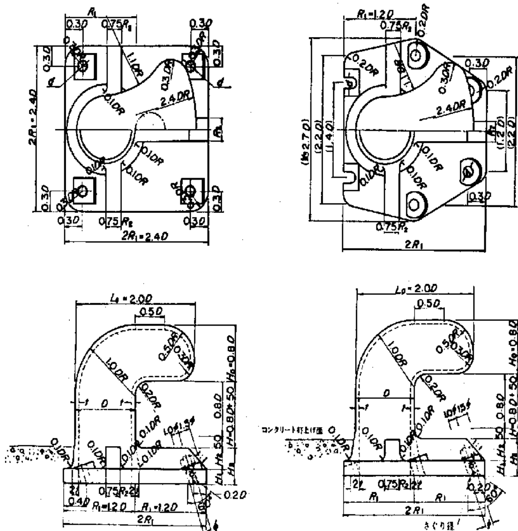
設計けん引力が 35, 50, 70, 100 トンの場合
