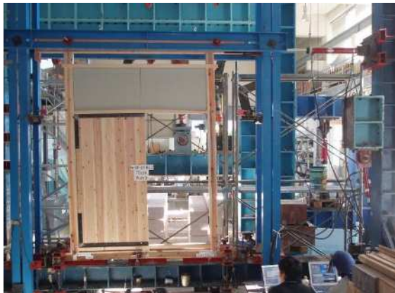
耐震補強パネル水平加力実験
