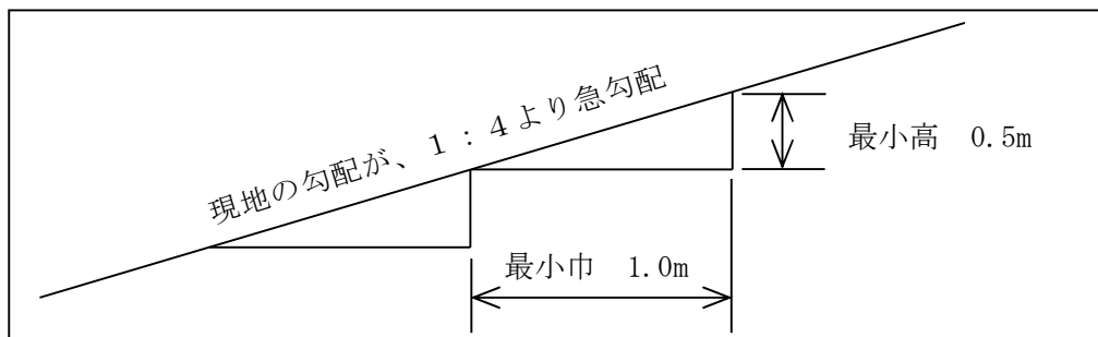
図 2-1 盛土基礎地盤の段切
