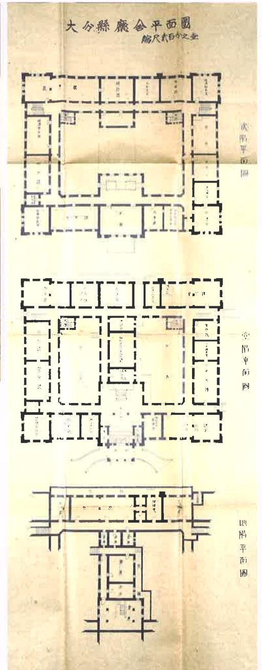
旧県庁舎平面図(『国有財産報告』)
