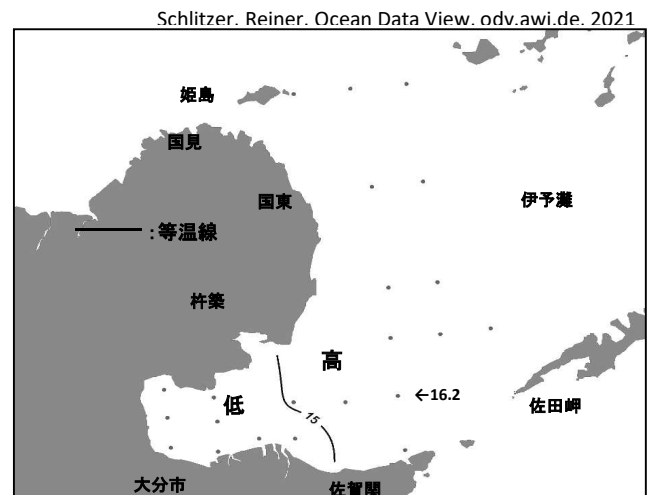
30層水温分布
