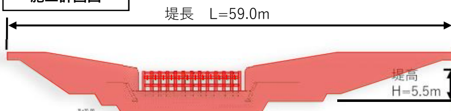
施工計画図
